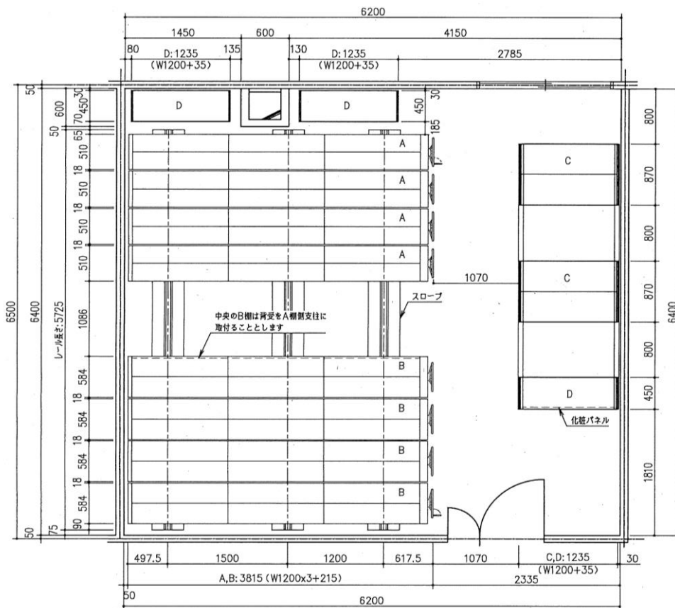
2階 倉庫 配置図 S=1/50
